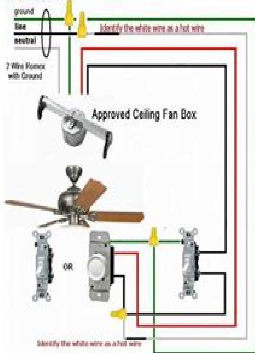
Ceiling Fan Wiring Diagram #2
