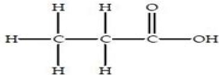
Struktur asam propionat
