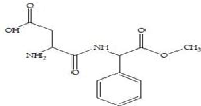
Struktur aspartam
