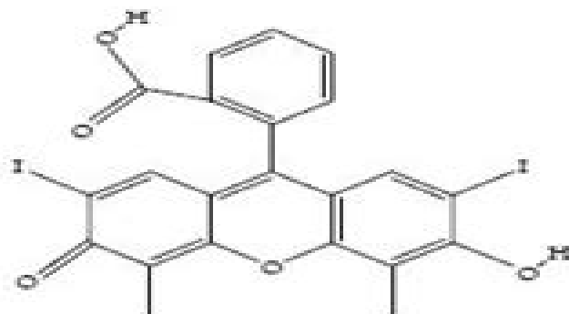
Struktur FCF
