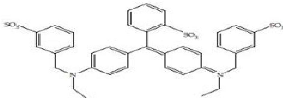
Struktur eritrosin
