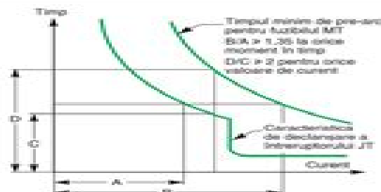
Fig. B118: Selectivitatea între fuzibile de MT și declanșarea întreruptorului JT, pentru protecția transformatorului.
