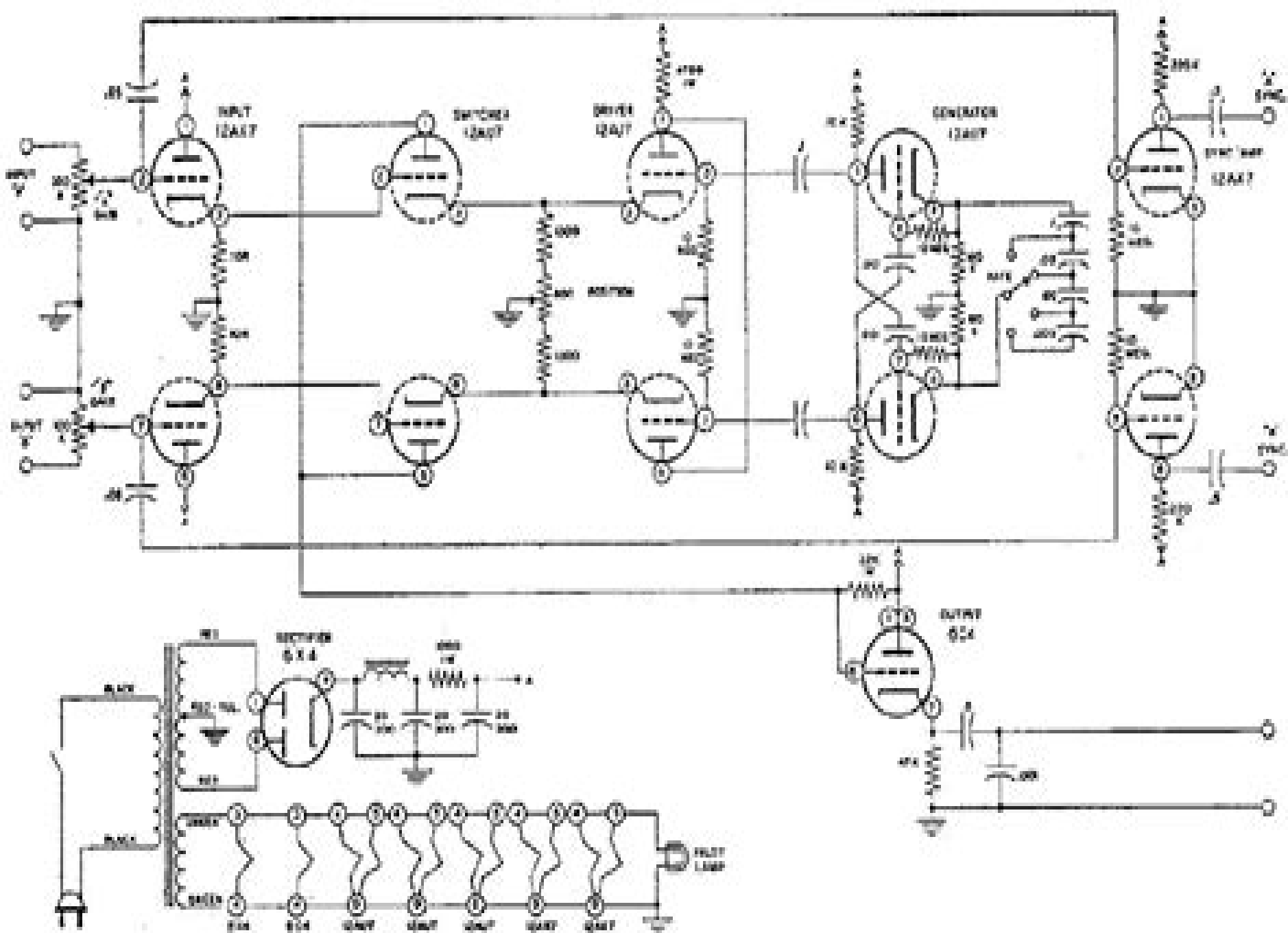
Schema del commutatore elettronico Heath 83.
