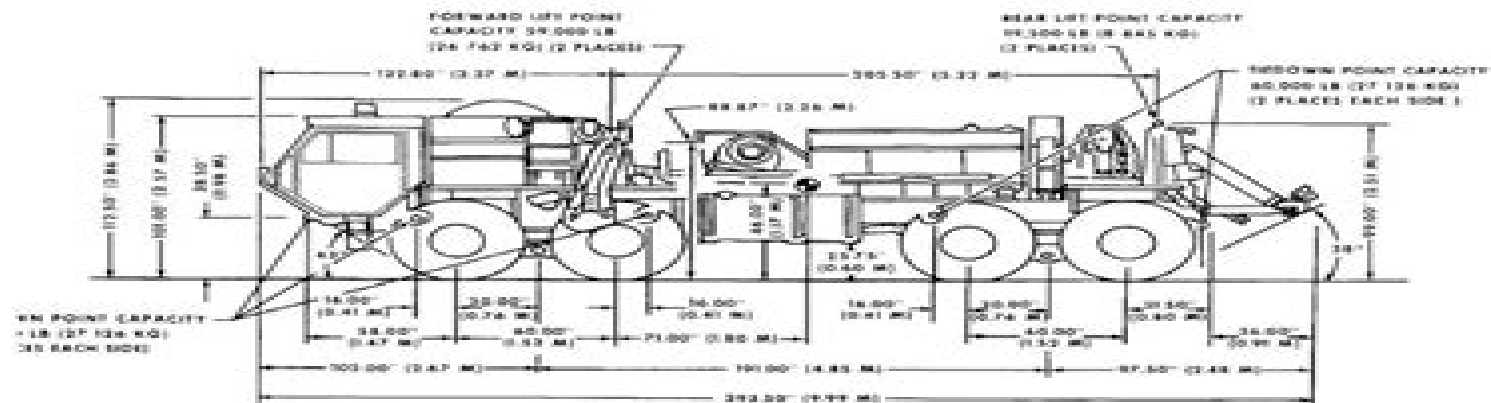
LEFT-SIDE ELEVATION
