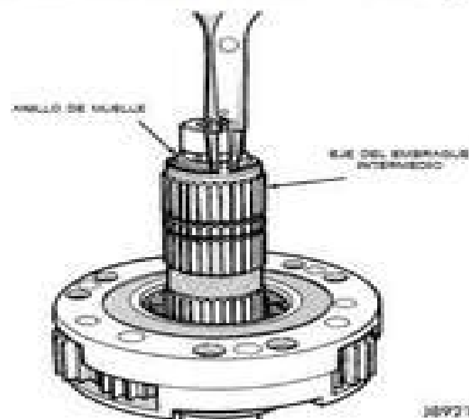
Fig. 76 Instalación del anillo de muelle del eje del embrague
