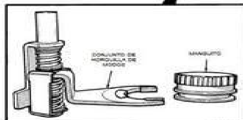
Fig. 78 Instalación de la horquilla y manguito de modos
