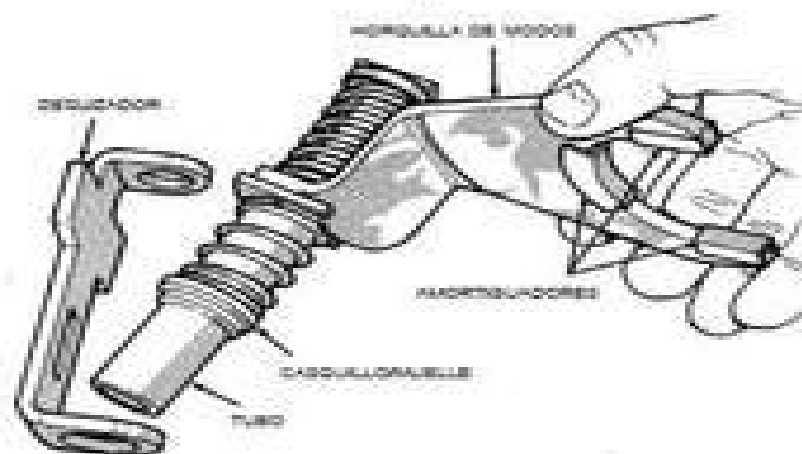
Fig. 76 Instalación del anillo de muelle del eje del embrague
