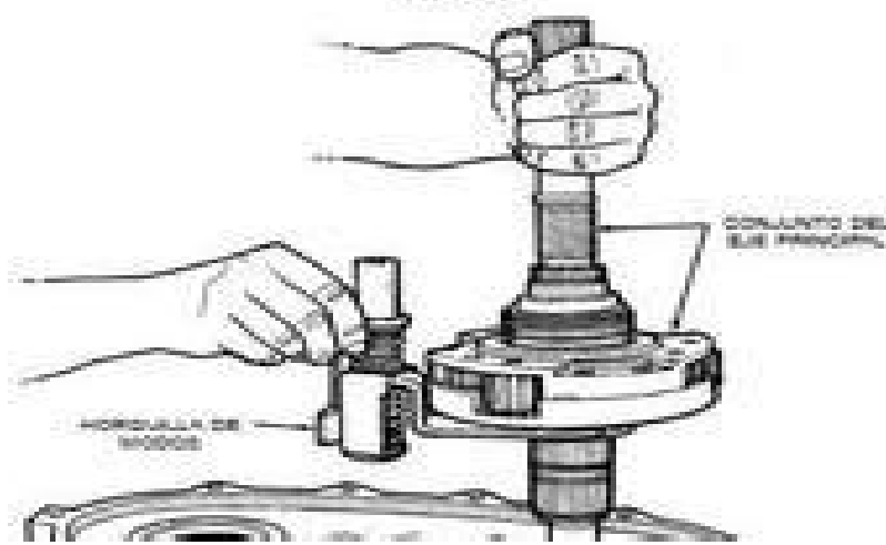
Fig. 78 Instalación de la horquilla y manguito de modos
