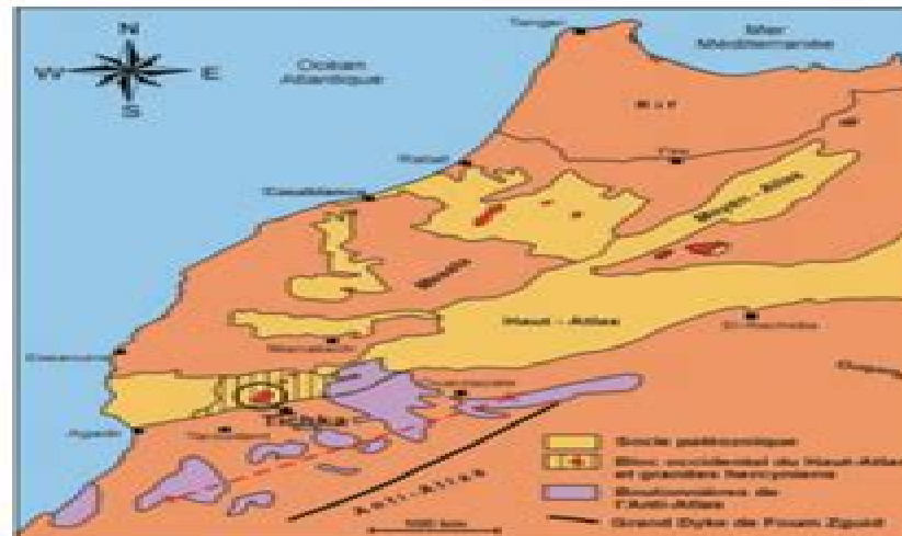
Fig 1.1: Situation géographique et géologique du Massif du Tichka En traitillé rouge, coupe présentée à la fig 7.2b. A,B,C : localisation des logs présentés en annexe II .
