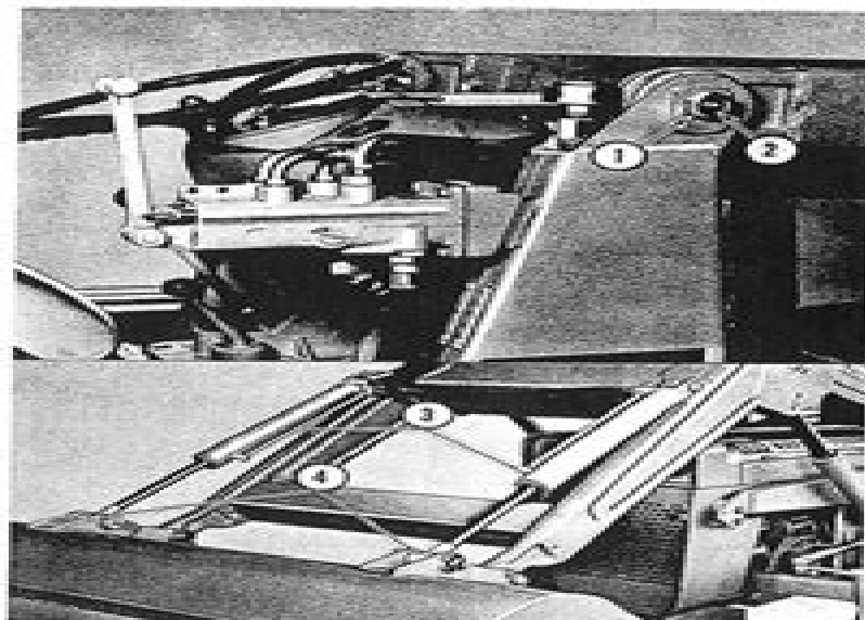
Fig. 12 - Lubrication Points
