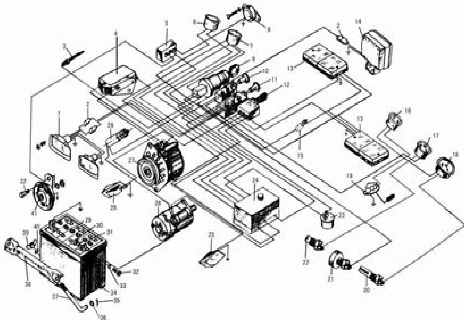
图 16 电器系统 (组合型)
