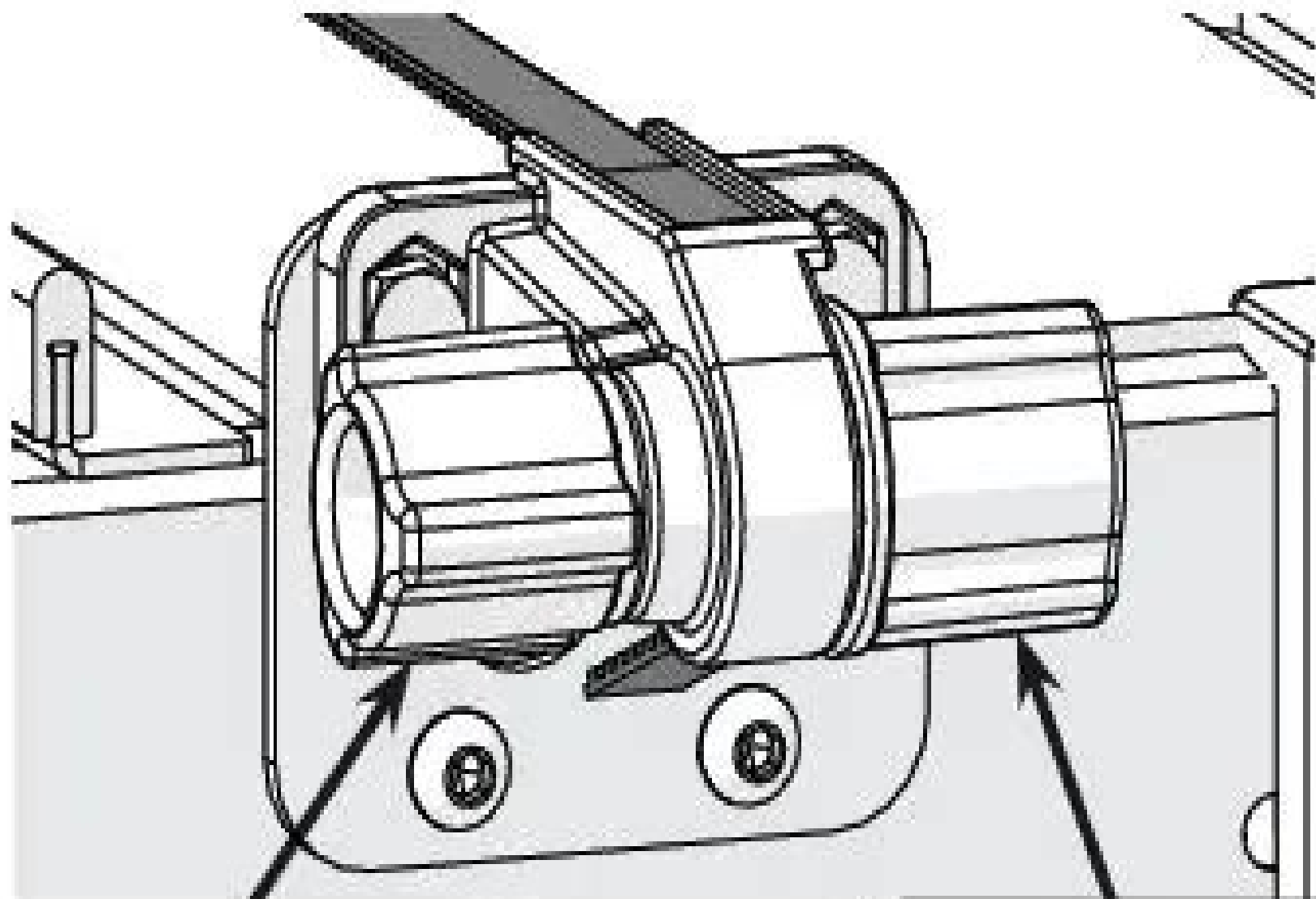
Ratchet Knob
