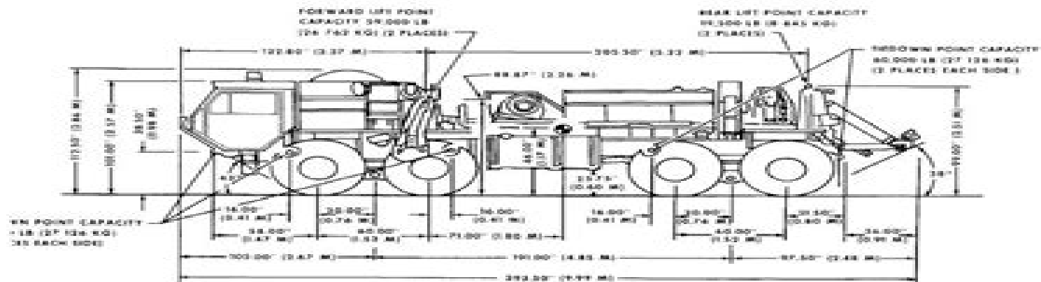
LEFT-SIDE ELEVATION
