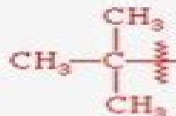
tert-butyl
