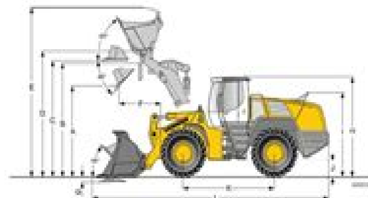
Fig. 28 Dimensions
