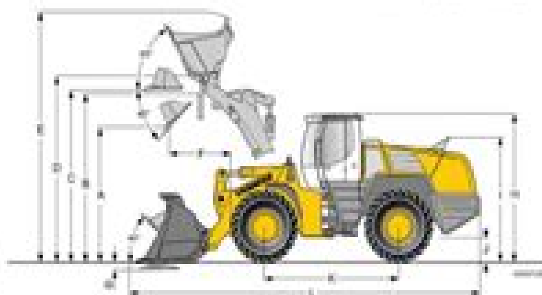
Fig. 20 Dimensions
