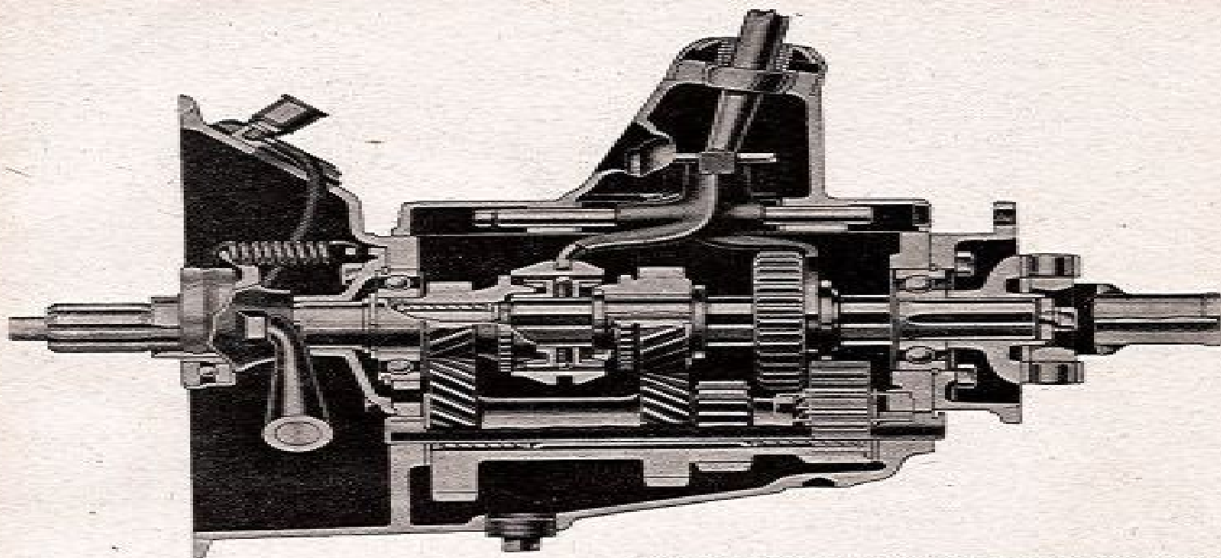
Fig. 39. Doorsnede van een synchro-mesh gangwissel.
