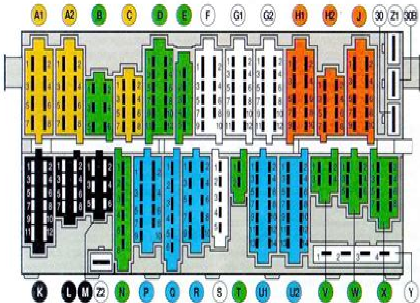
Рис. 3. Схема расположения разъемов в монтажном блоке
