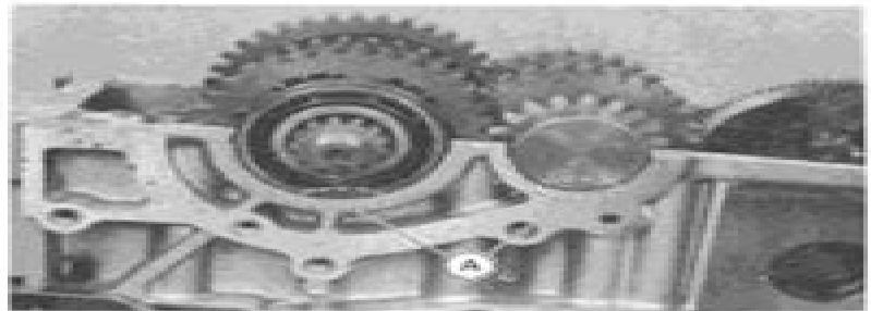
A. No clearance
