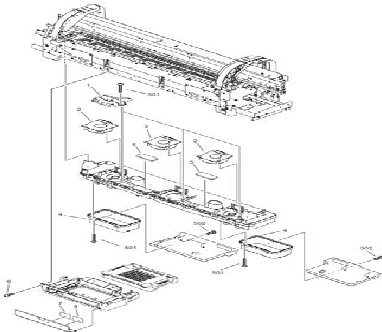
FIGURE 08 AIR FLOW FAN UNIT
