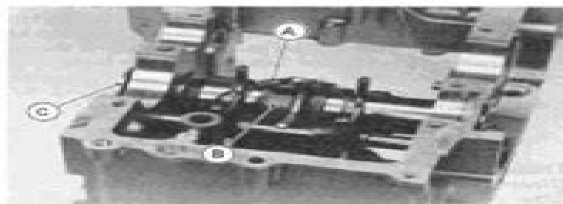
A. Cotter pin B. Long end C. Pin plate
