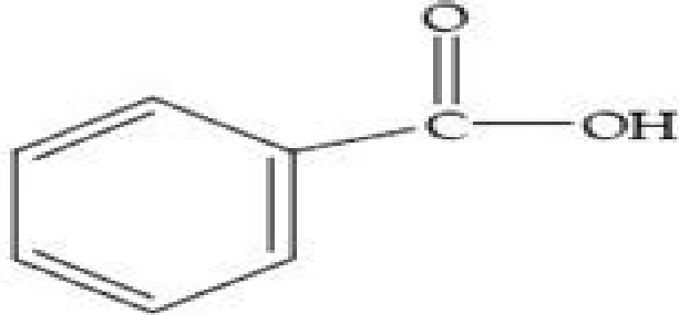
Struktur asam benzoat
