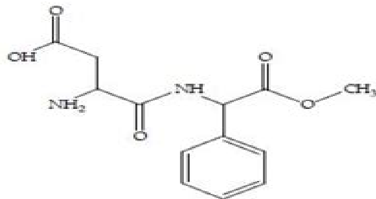
Struktur aspartam
