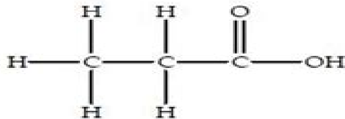
Struktur asam propionat
