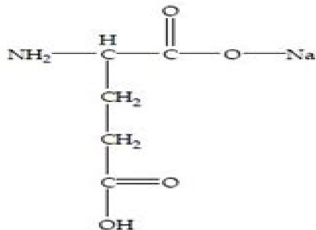
Struktur MSG ( Monosodium glutamate )
