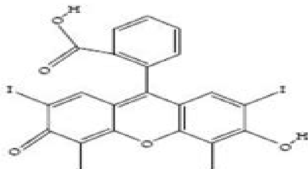
Struktur FCF
