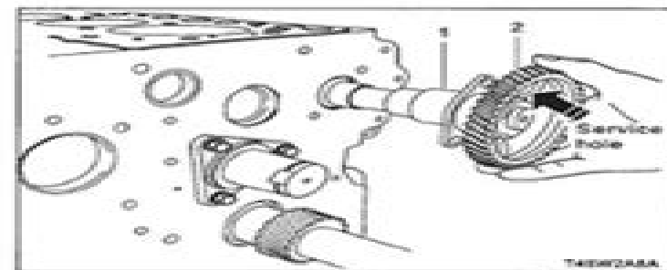
(1) Camshaft
