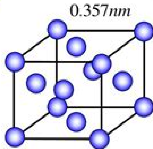
\gamma -Fe austenite FCC
