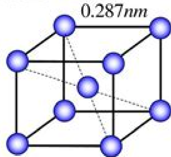
\alpha -Fe ferrite BCC
